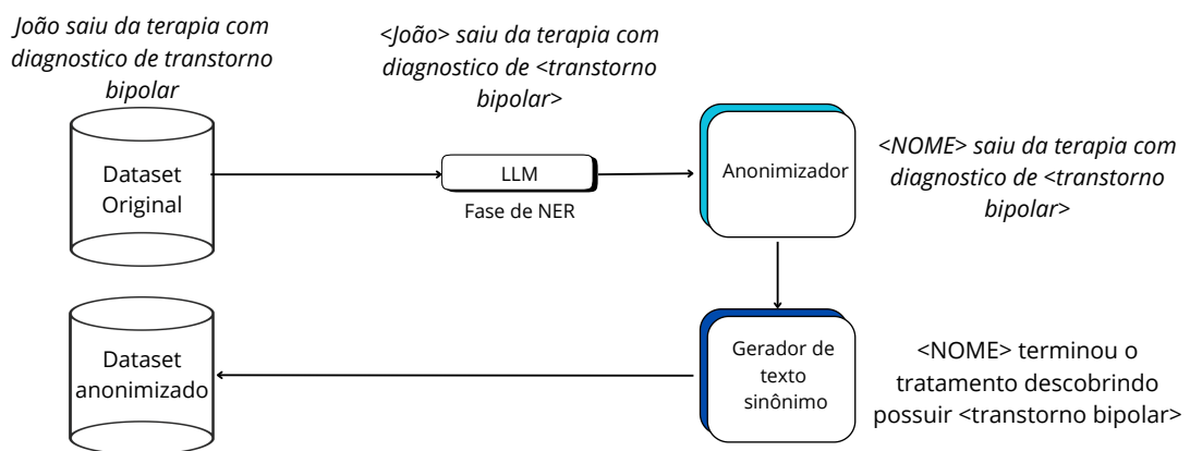
Figura 5.1: Pipeline do processo de anonimização.
